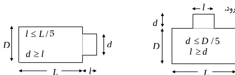
ابعاد پیش‌آمدگی در طول ساختمان
