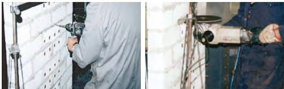
شکل ت-۲-۲ نحوه ایجاد شکاف دایره‌ای و مستطیلی
