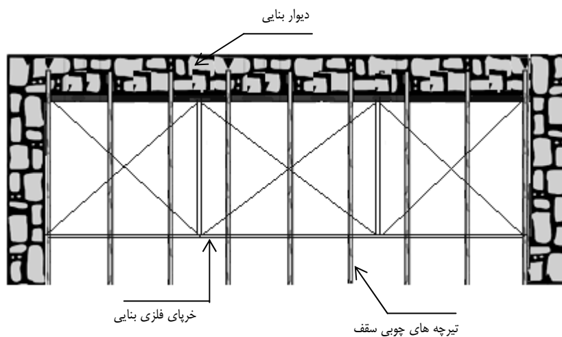
شکل ت-۵-۲۳ تأمین یکپارچگی سقف با استفاده از خرباهای افقی
