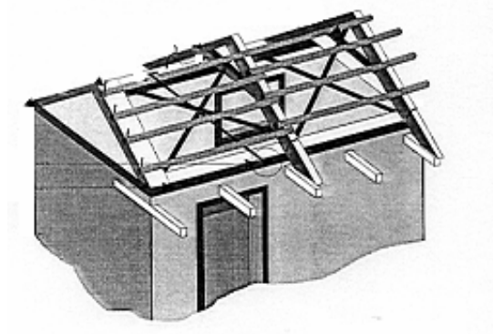
شکل (ت-۵-۲۴) یکپارچگی سقف‌های شیبدار
