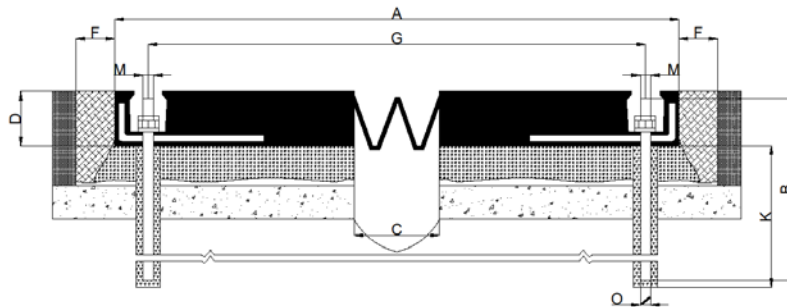
جزئیات درز انبساط تیپ W
