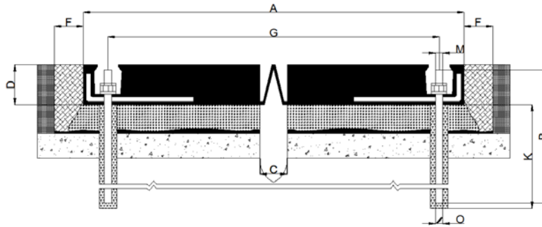
جزئیات درز انبساط تیپ V
